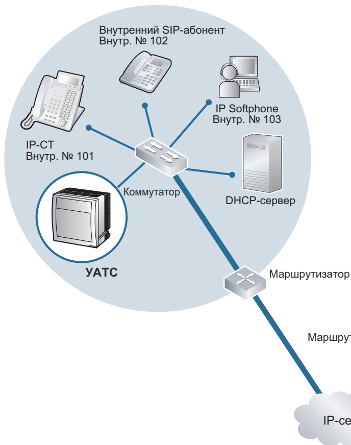
Локальная сеть центрального офиса
